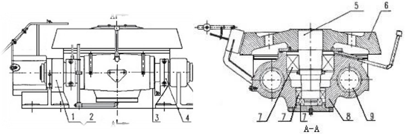
图 1 挡轮的结构图
